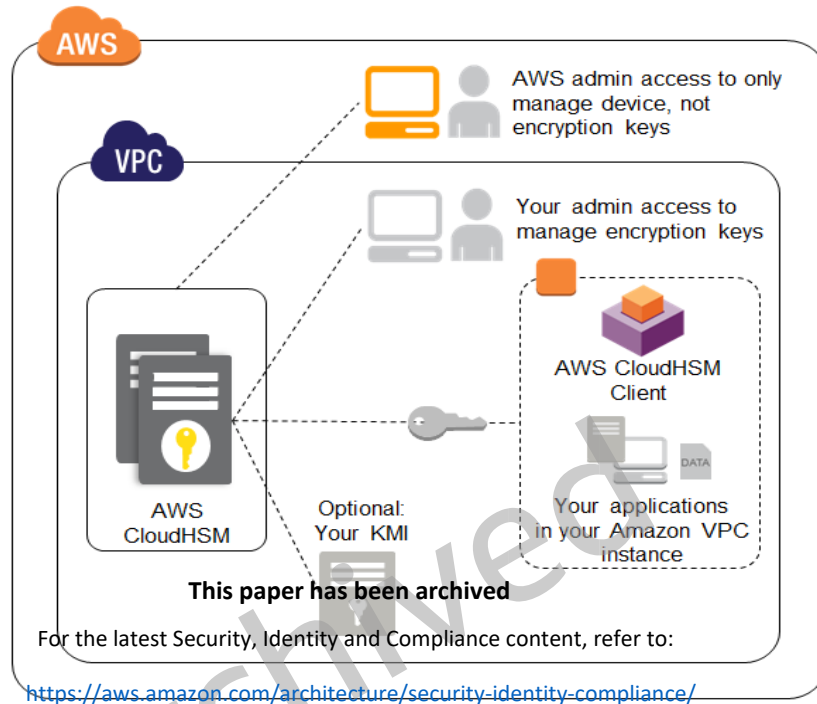
그림 7: Amazon VPC에 배포된 AWS CloudHSM
