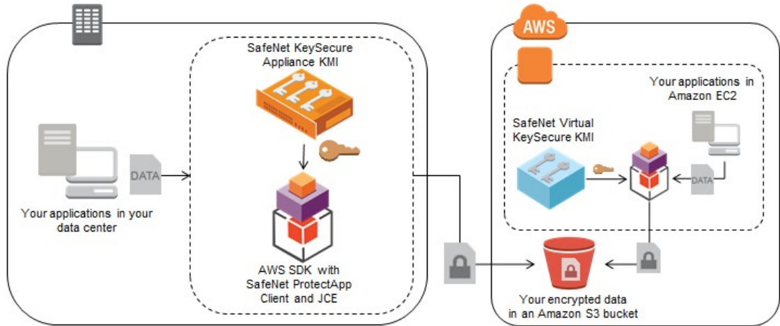
그림 3: SafeNet ProtectApp 및 SafeNet KeySecure KMI를 사용하여 온프레미스 시스템 또는 Amazon EC2의 애플리케이션 내에서 Amazon S3 클라이언트 측 암호화
