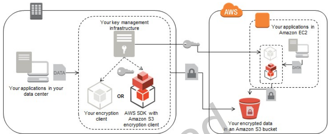
그림 2: 온프레미스 시스템 또는 Amazon EC2 애플리케이션 내에서 Amazon S3 클라이언트 측 암호화
