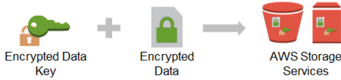
그림 8: 봉투 암호화
