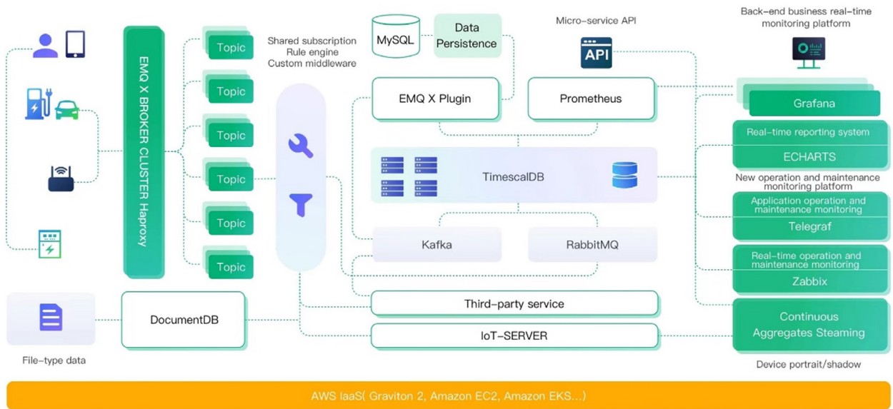
EMQ 云边一体化充电桩运营解决方案参考架构
