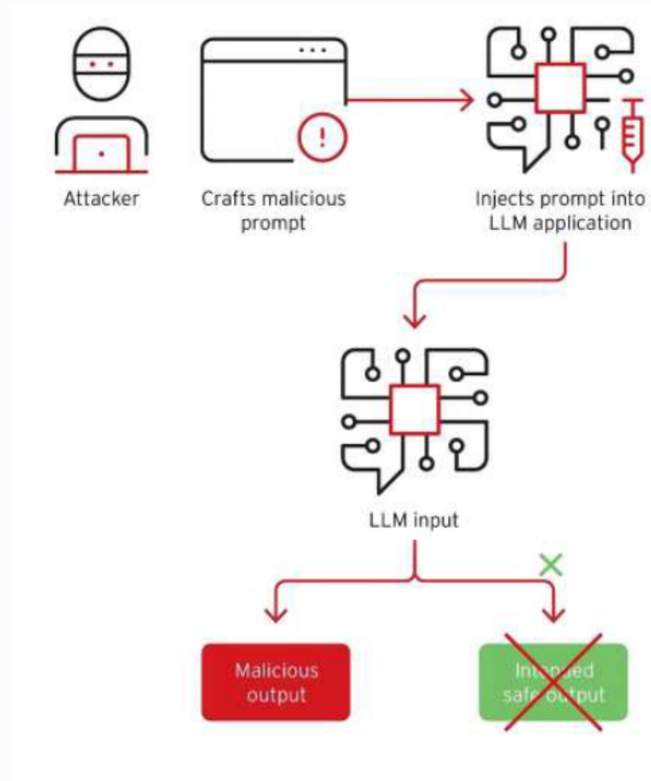
开源AI供应链攻击流程图 (图源：Trend Micro)
