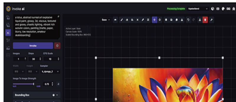
InvokeAI
